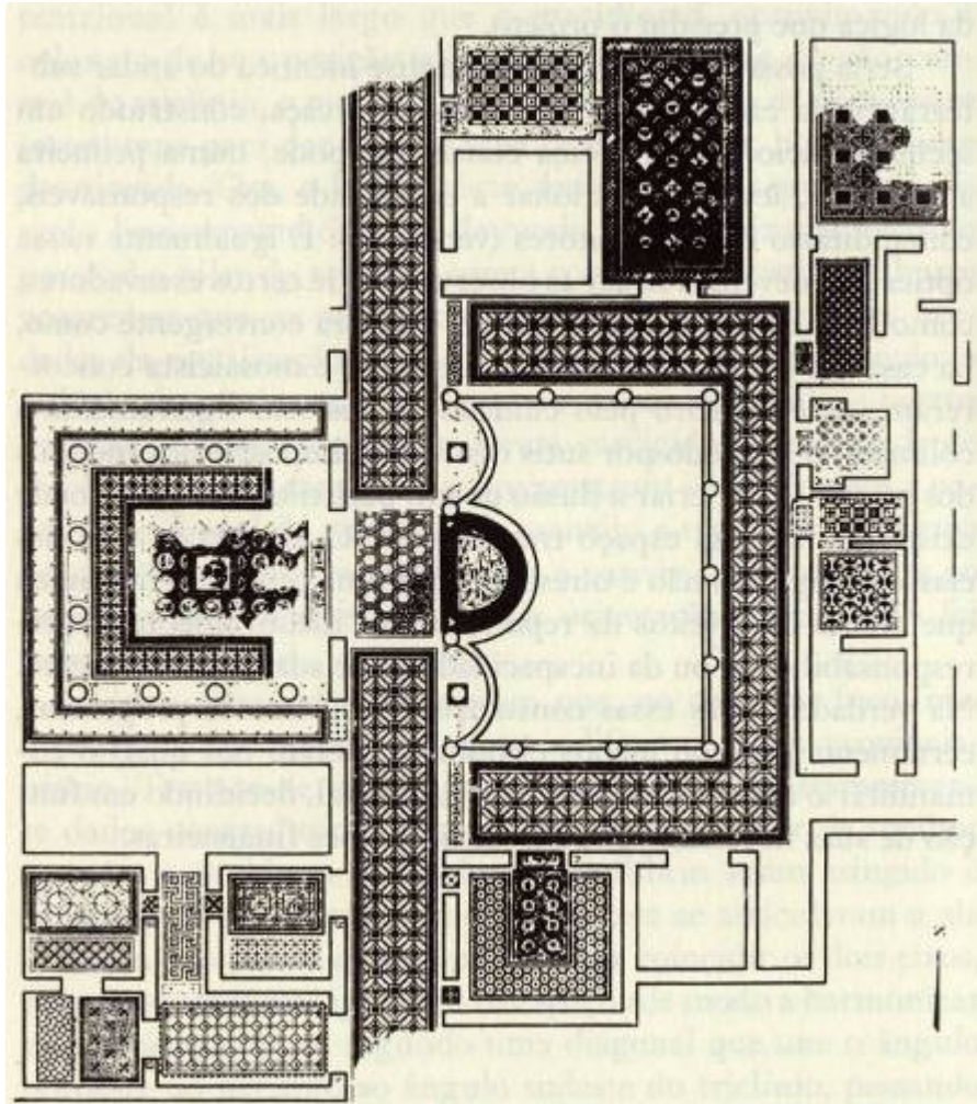
Figura 7. Acholla, casa de Netuno (S. Gozlan, Karthago , 16, 1971-2, fig. 2). Peristilo com oecus a oeste, triclinio ao sul e dormitórios servidos por antecâmaras ou corredores no ângulo sudoeste. Aqui devo agradecer a M. E. Vast, fotógrafo na UAV da ENS de Saint-Cloud, que me ajudou a organizar essa documentação. [pág. 330]
