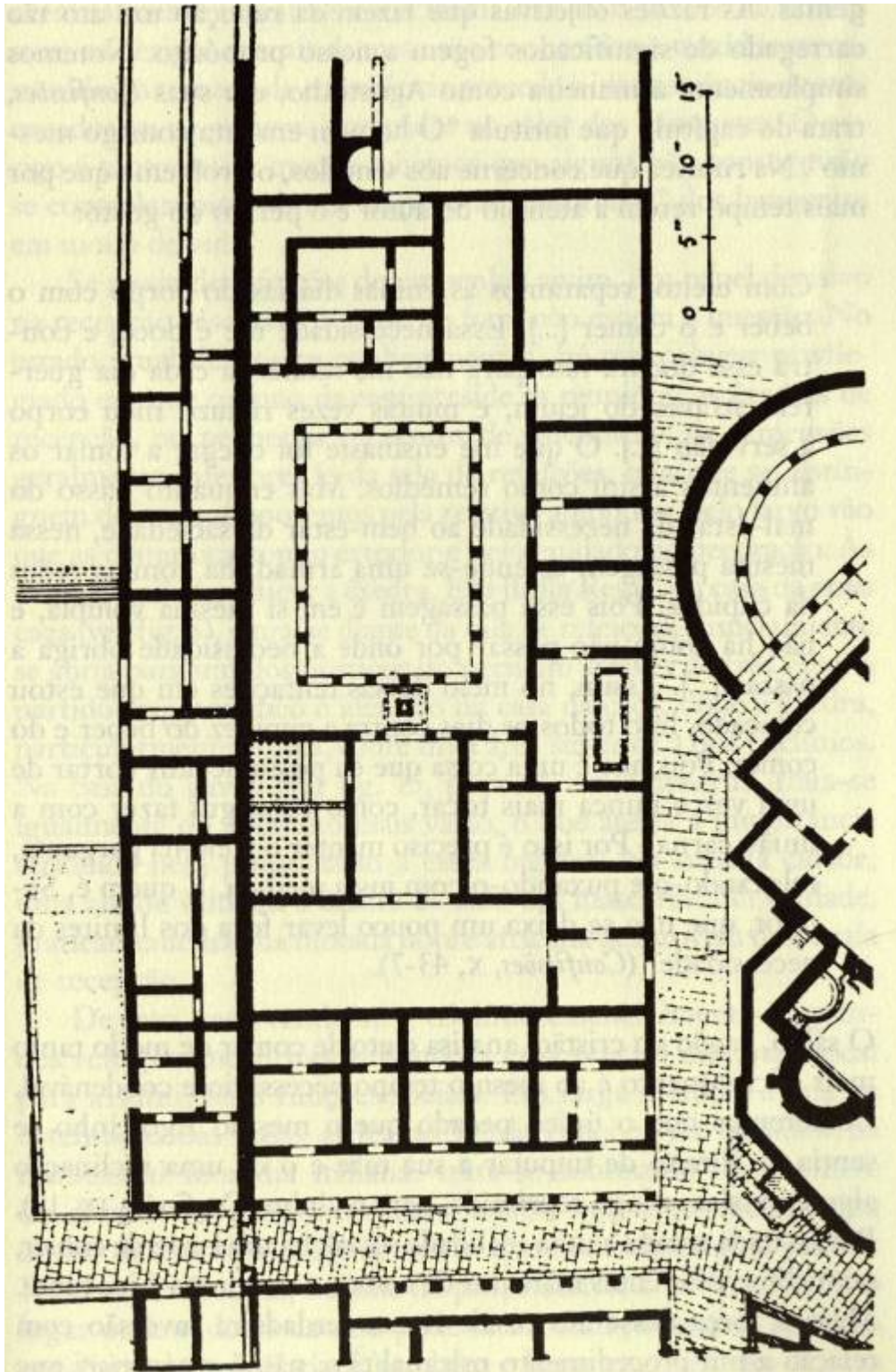
Figura 17 Timgad, casa do Hermafrodita. À esquerda, sob o pórtico que acompanha o cardo maximus que separa esta residência das de Sécio, fileira de lojas; depois, da esquerda para a direita, ou seja, em direção ao leste, vestíbulo de entrada dando para uma sala contígua a um grande aposento (11 x 7,60 m) aberta nas duas extremidades por três vãos: sem dúvida trata-se do triclínio. A espessa parede que delimita a casa ao norte corresponde ao traçado da primitiva muralha.
