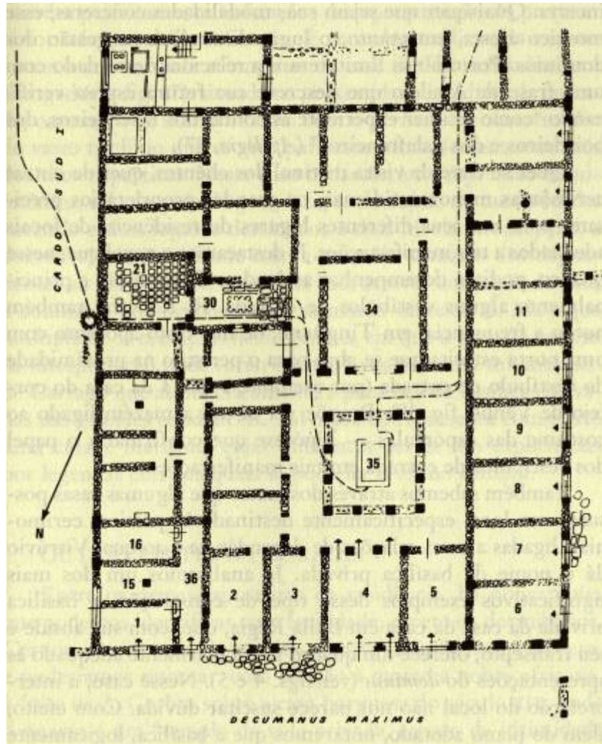
Figura 20. Volubilis, casa da moeda de ouro (Étienne, ibid , pr. x). Esta moradia, uma das mais vastas de Volubilis, ocupa mais de 1700 metros quadrados. Plano quase axial. 1, 15, 16 e 36: apartamento independente; 4: vestíbulo (6 x 5 m); 2, 3 e 5: lojas comunicando-se com a casa; 6 a 11: lojas independentes; 35: peristilo quadrado (12,50 m); 34: triclinio (?) (7,40 x 6,50 m) com duas pequenas portas de serviço; 30: pátio secundário com tanque comunicando-se em particular com a peça 21 (5,60 x 4,30 m) com piso de mármore. Ao sul, fora do plano, estende-se um vasto setor econômico compreendendo uma fábrica de azeite e uma padaria. [pág. 367]
